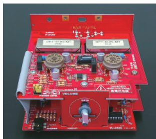
組み立ての完了した基板ユニット
